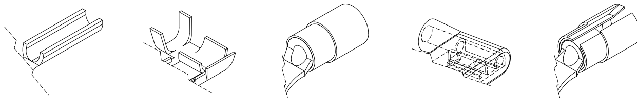
COLLETTO APERTO OPEN BARREL
